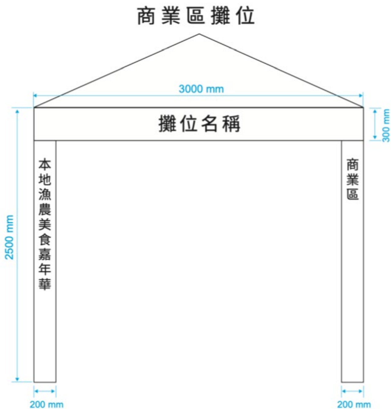
圖(二) 標準商業區攤位圖
